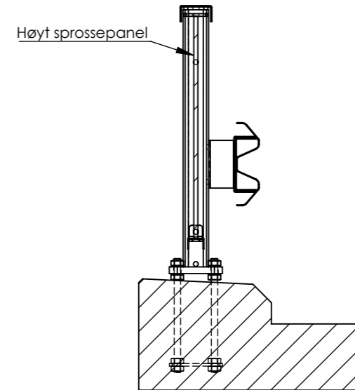
SECTION D-D SCALE 1 : 20
